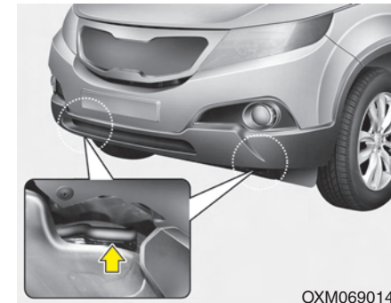
Крюк для крепления к платформе (для буксировки на эвакуаторе, при наличии)
